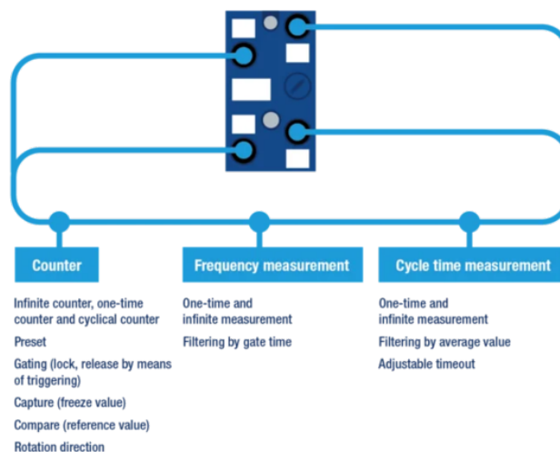
Afb.: Door de vele functies en de twee of vier afzonderlijk instelbare metingen kunt u met de flexibele ASi-5-telmodules voordelig een scala aan toepassingen gebruiken.
