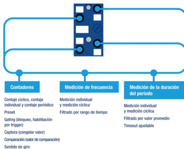
Fig.: Gracias a sus numerosas funciones y a las variantes de 2 o 4 entradas de contador configurables, los nuevos módulos de contaje ASi-5 proporcionan flexibilidad para solucionar de forma económica, las aplicaciones más diversas.
