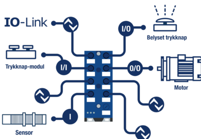
Fig.: Takket være de fleksible konfigurationsmuligheder med portene kræves der ingen yderligere standard-digitalmoduler – som det her ses ved 8-port IO-Link Master BWU4386 .
