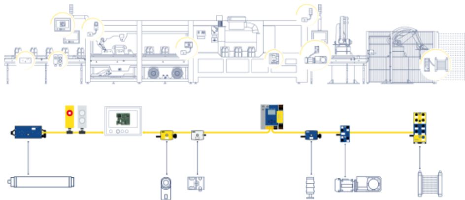
Fig.: ASi o ASi-5 consente di integrare un'ampia gamma di dispositivi IO-Link, soluzioni di azionamento e interruttori di sicurezza, nonché altri sensori e attuatori sicuri.
