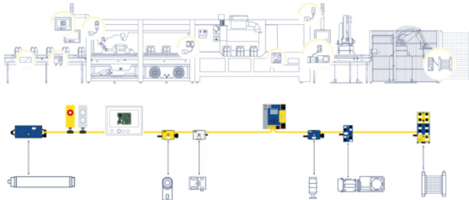
Fig.: ASi o ASi-5 permite integrar una amplia gama de dispositivos IO-Link, soluciones para accionamientos e interruptores de seguridad, así como otros sensores y actuadores seguros.
